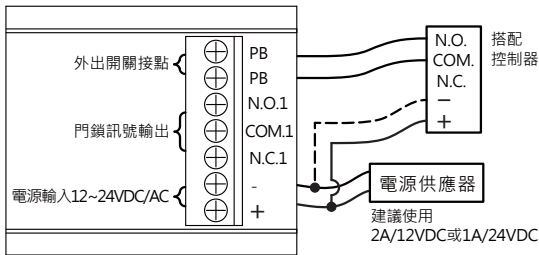
圖A 為PBH-100M-SO系列控制器接線圖
