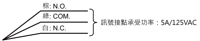
圖B 為PBH-110M-ME系列訊號接線圖
