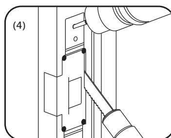
依照貼紙標線範圍切孔、鑽孔。 注意:半埋式與全埋式安裝切孔 範圍不同
