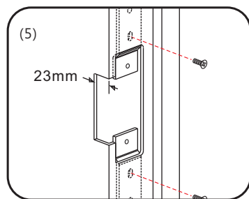
鎖上固定墊片
