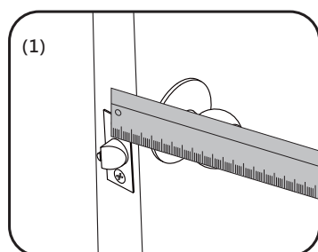
測量喇叭鎖舌的深度位置
