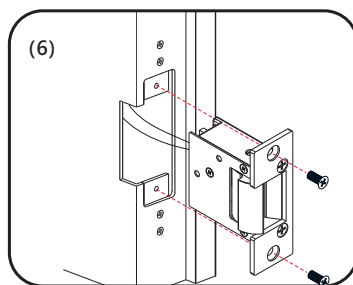
接上電源線，固定陰極鎖後 進行測試。
