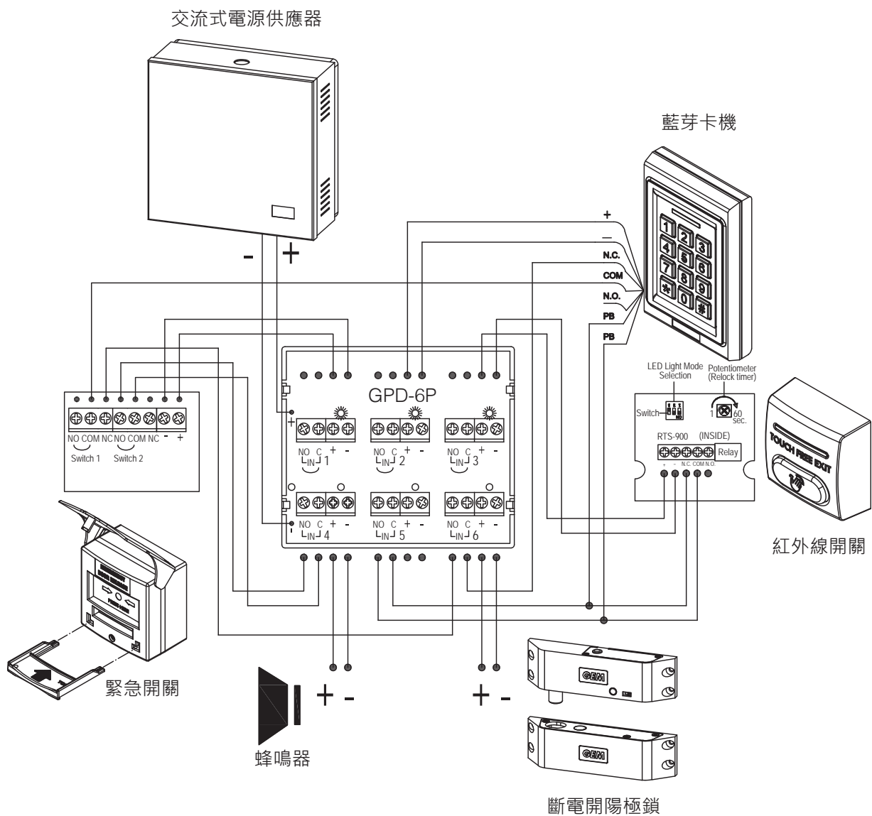
電壓分流版接線圖
