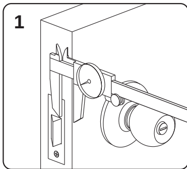
測量機械鎖舌的深度位置
