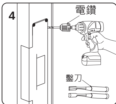
依照貼紙標線範圍切孔、鑽孔(注意：半埋式與埋式的切孔範圍不同)
