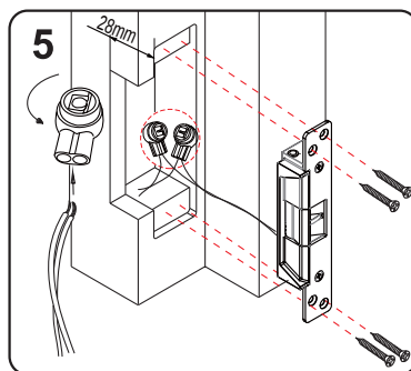
接上電源線，固定陰極鎖，進行測試。
