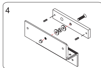
4 依照圖示組合吸附板以及"Z"型輔助架(橡膠墊片務必加入)。
