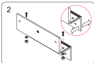
2 組裝輔助架。必須注意輔助架可以調動。
