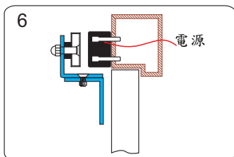
6 吸附板組與電磁鎖正確的吸住後...
