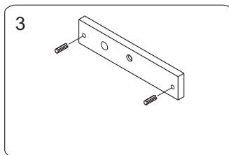
3 把插杓輕輕敲入吸附板。其目的是防止吸附板轉動。
