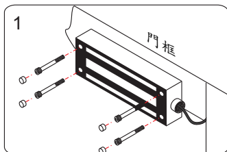
1 在門框適當位置直接固定電磁鎖。必須注意不可影響門扇的開關。
