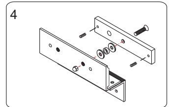
把插枱輕輕敲入吸附板。其目的是防止吸附板轉動。
