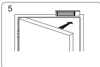
依照圖示組合吸附板以及"Z"型輔助架(橡膠墊片務必加入)。
