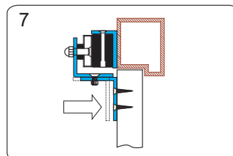
吸附板組與電磁鎖正確的吸住後，調整Z型輔助架部分頂到門扇。
