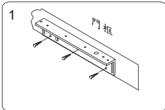
在門框適當位置固定LZ型輔助架的L架部分。必須注意不可影響門扇的開關。
