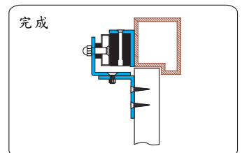
鎖緊Z型輔助架，完成。
