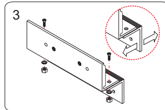
組裝LZ型輔助架的Z架部分。必須注意輔助架可以調動。
