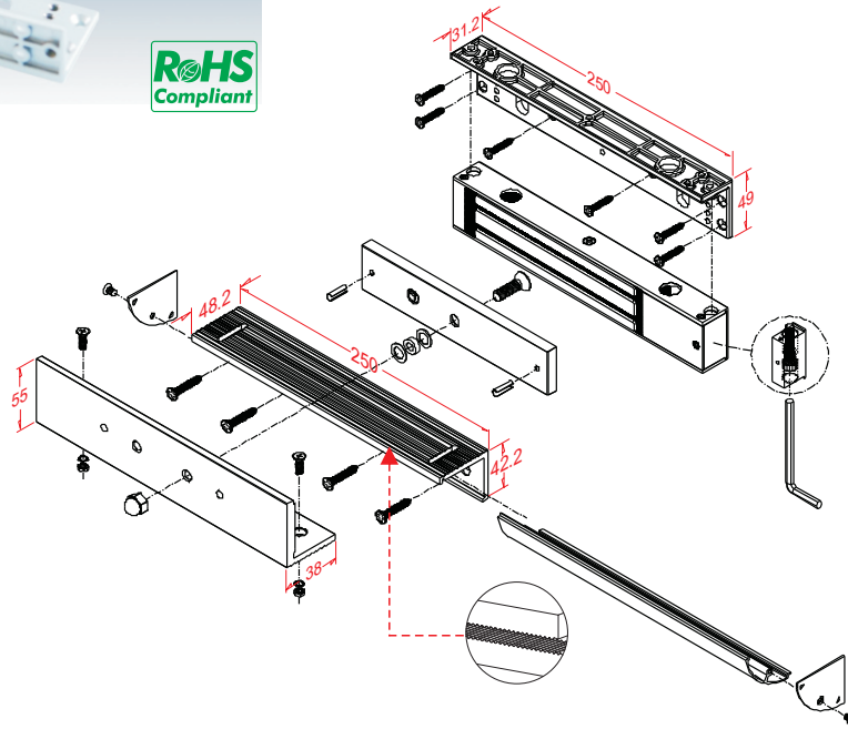
運用的電磁鎖型號:GEM-600 系列
