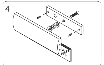
4 把插枓輕輕敲入吸附板。其目的是防止吸附板轉動。
