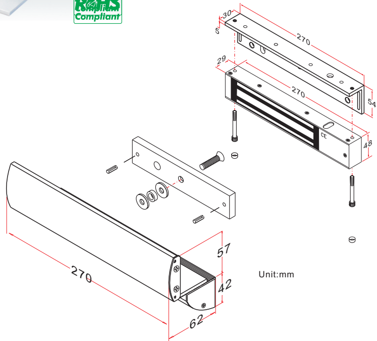
運用的電磁鎖型號: EM-350 系列
