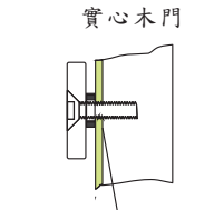
門內先鑽6.8mm孔金屬板攻M81.25mm的螺絲牙
