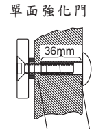
單面強化門 先鑽8mm孔貫穿門扇再從門外側擴大為12.7mm孔，深度為36mm
