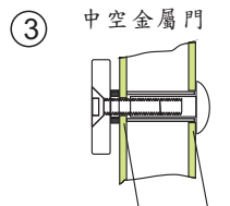
中空金屬門 先鑽8mm孔貫穿門扇再從門外側擴大為12.7mm孔
