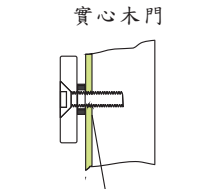
實心木門 門內先鑽6.8mm孔金屬板攻M81.25mm的螺絲牙
