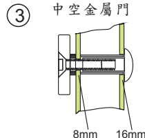
先鑽8mm孔貫穿門扇再從門外側擴大為12.7mm孔
