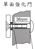
先鑽8mm孔貫穿門扇再從門外側擴大為12.7mm孔，深度為36mm
