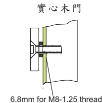
門內先鑽6.8mm孔再從門外側擴大為12.7mm孔，深度為36mm
