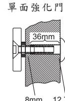
先鑽8mm孔貫穿門扇再從門外側擴大為12.7mm孔，深度為36mm
