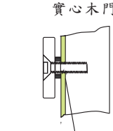
門內先鑽6.8mm孔金屬板攻M81.25mm的螺絲牙
