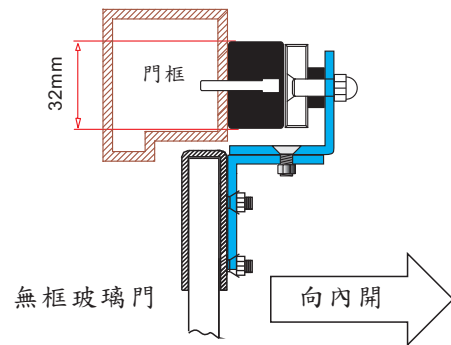
10003F電磁鎖(正面孔)安裝示意圖
