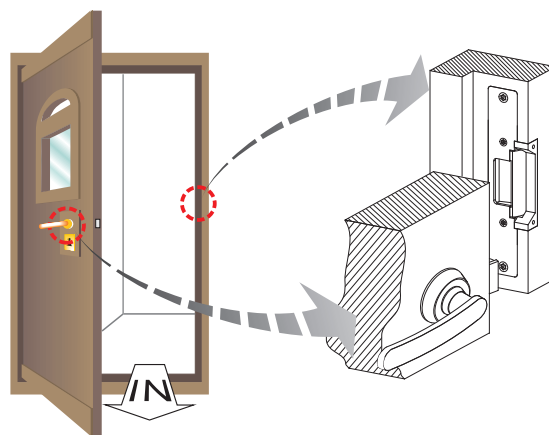
GK350-1224 木門框外露式安裝示意圖
