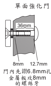
先鑽8mm孔貫穿門扇再從門外側擴大為12.7mm孔，深度為36mm
