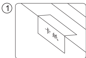
安裝卡紙沿虛線折成直角
