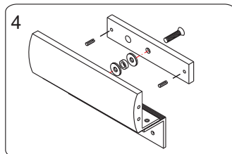
4 把插桿輕輕敲入吸附板。其目的是防止吸附板轉動。
