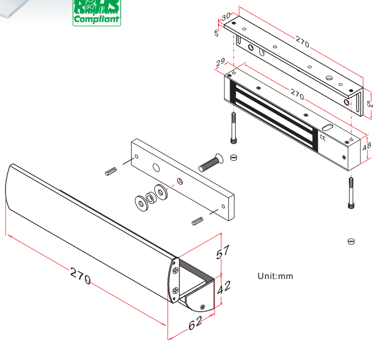
運用的電磁鎖型號: EM-350 系列
