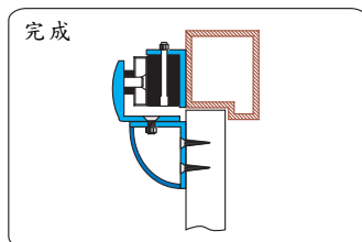
8 鎖緊Z型輔助架，完成。
