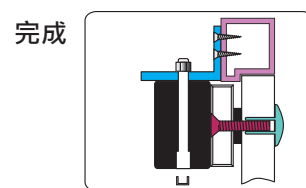
測試無誤後蓋上塞頭
