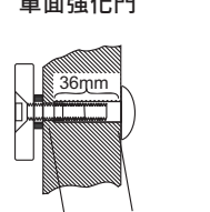
單面強化門 先鑽8mm孔貫穿門扇，再從門外側擴大為12.7mm孔，深度為36mm
