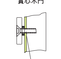
實心木門 門內先鑽6.8mm孔，金屬板攻M8-1.25mm的螺絲牙
