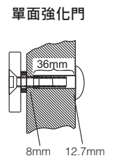
先鑽8mm孔貫穿門扇，再從門外側擴大為12.7mm孔，深度為36mm
