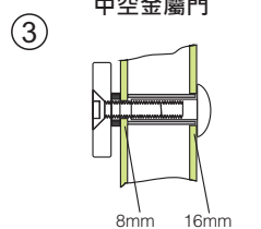
中空金屬門 先鑽8mm孔貫穿門扇，再從門外側擴大為12.7mm孔
