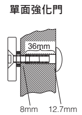
單面強化門 先鑽8mm孔貫穿門扇，再從門外側擴大為12.7mm孔，深度為36mm
