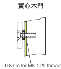
實心木門 門內先鑽6.8mm孔，金屬板攻M81.25mm的螺絲牙
