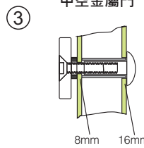
中空金屬門 先鑽8mm孔貫穿門扇，再從門外側擴大為12.7mm孔
