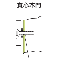
實心木門 門內先鑽6.8mm孔，金屬板攻M81.25mm的螺絲牙
