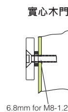
門內先鑽6.8mm孔，金屬板攻M8.1.25mm的螺絲牙
